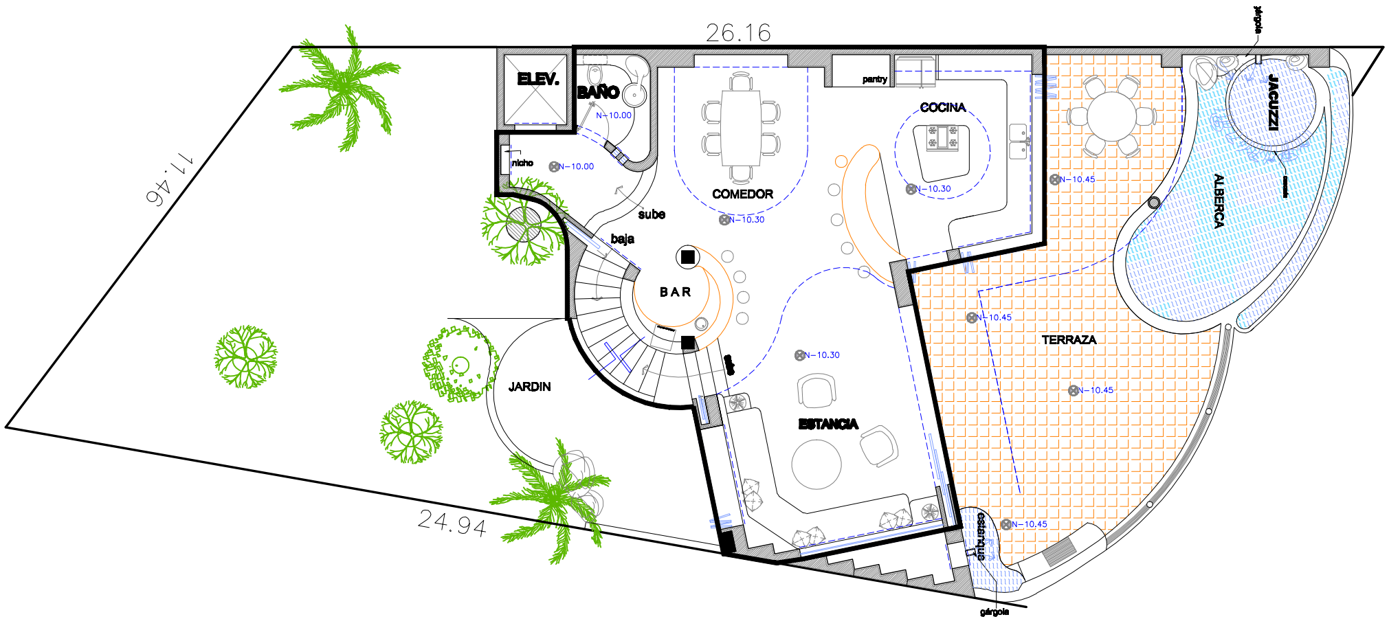
PLANTA NIVEL - 3 N-10.00 Escala 1: 100
